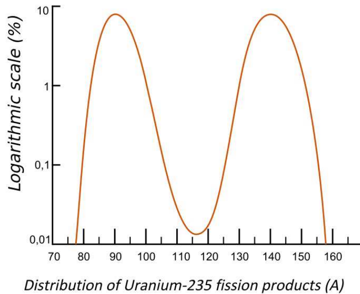
Abb. 32 Massenzahlverteilung der Spaltprodukte bei der Uranspaltung (Quelle: Wikimedia-Commons; das Bild unterliegt der License CC BY-SA 3.0; der Autor ist Mubs)
